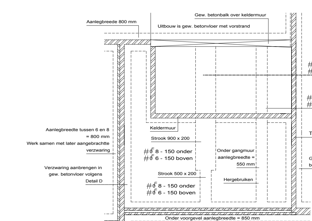
Schema funderingaanpassingen
