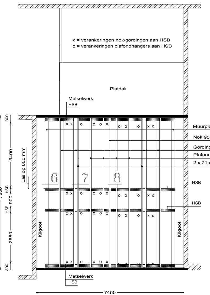
Kapplan/plafondhangers
