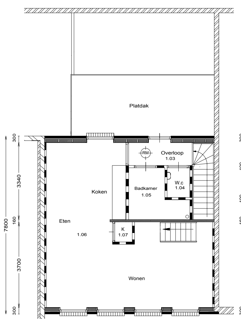
1e verdieping gewijzigd
