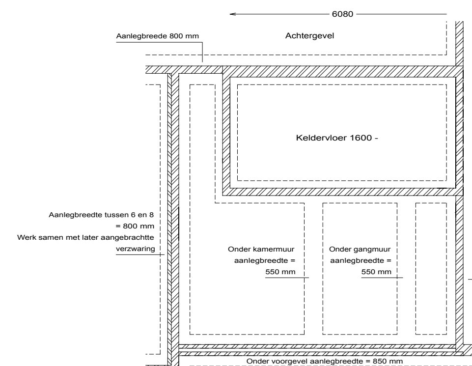
Schema bestaande funderingen
