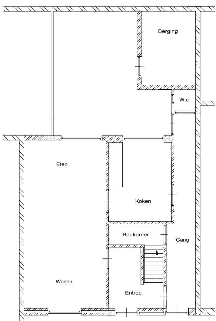
Plattegrond bestaand
