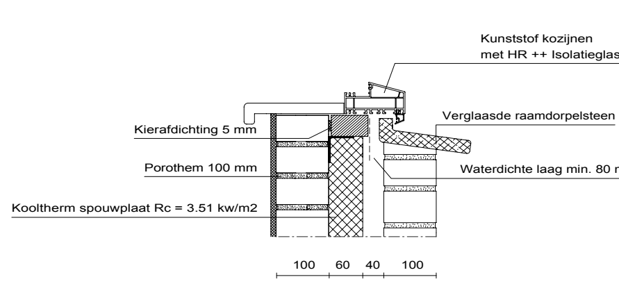
Aansluiting onderdorpel
