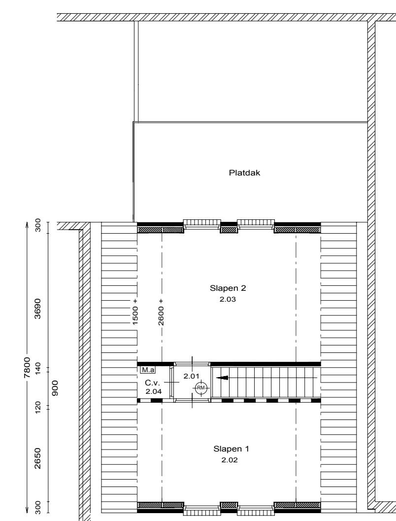
2e verdieping nieuw
