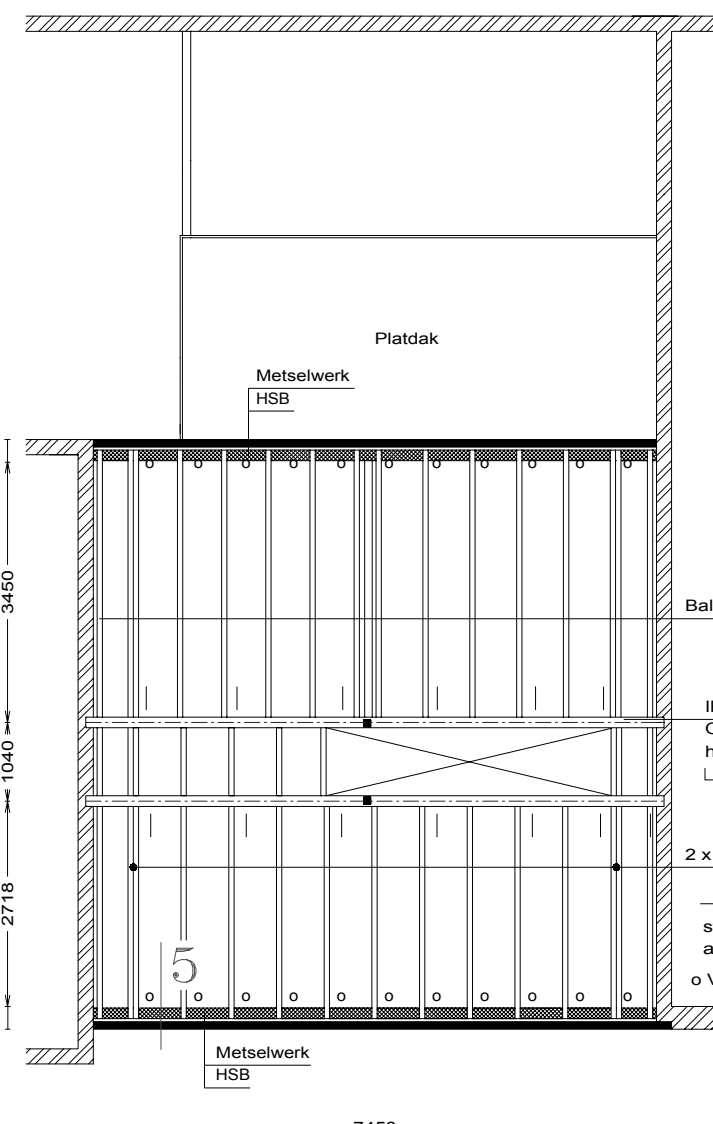
Balklaag 2e verd.
