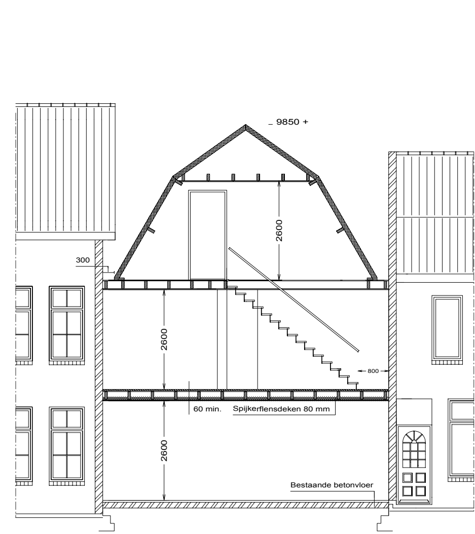
Algemeen dwarsdoorsnede
