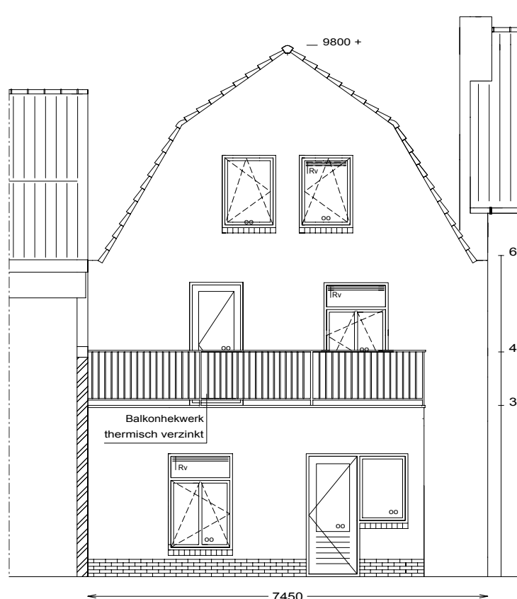
Achtergevel gewijzigd
