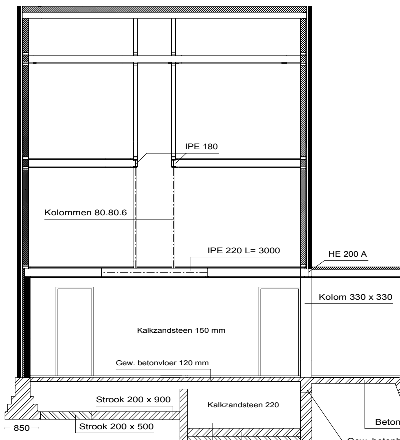
Schema constructieve dwarsdoorsnede
