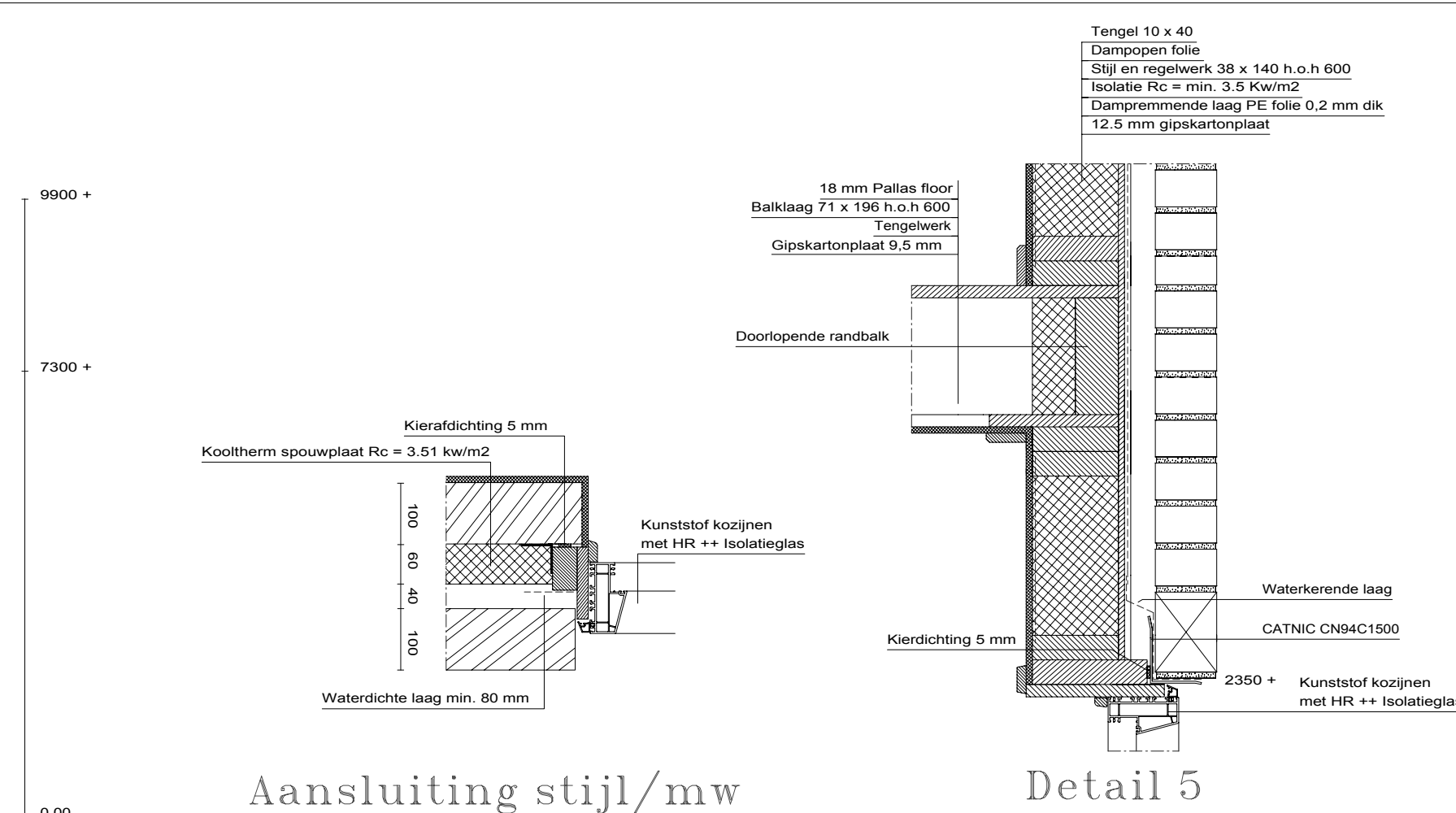
Aansluiting stijl/mw
