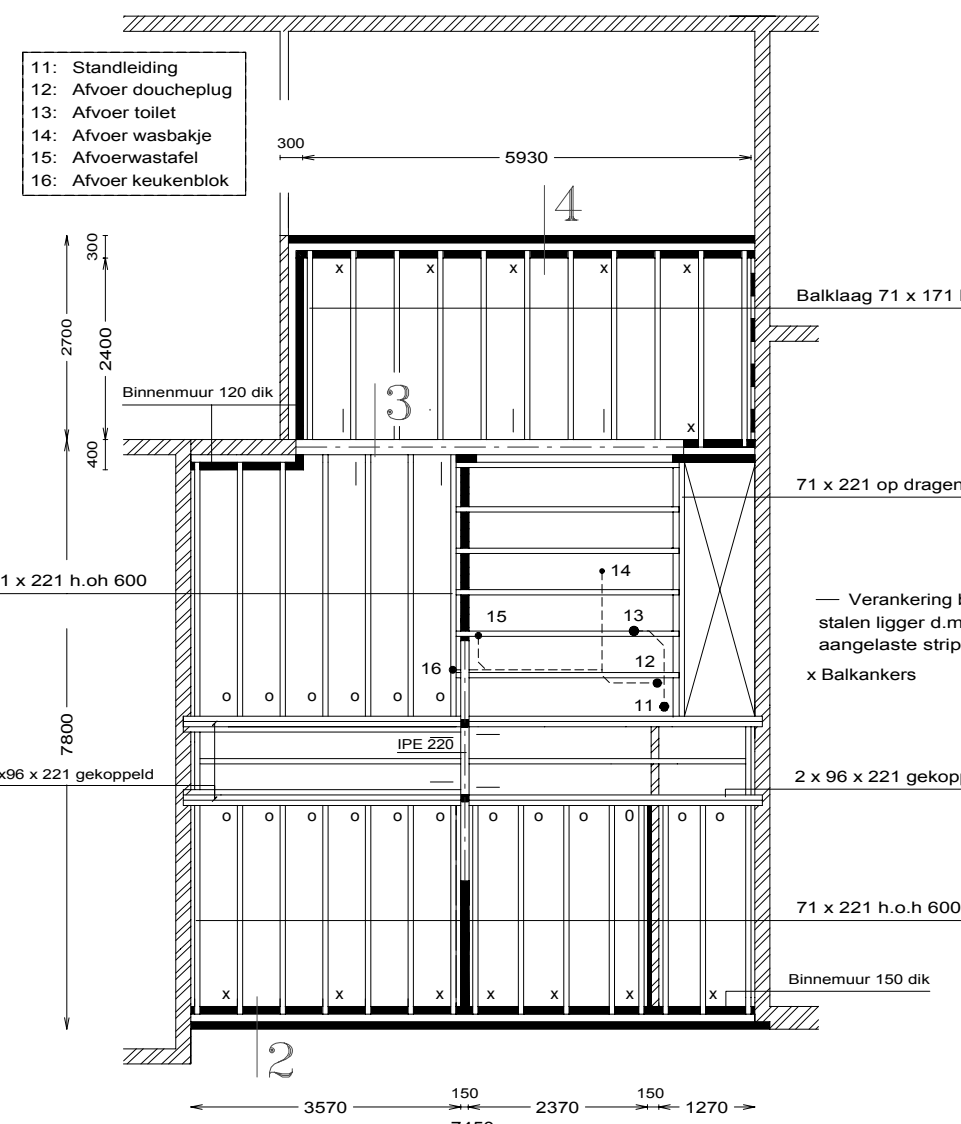
Balklaag/Riolering 1e verd.
