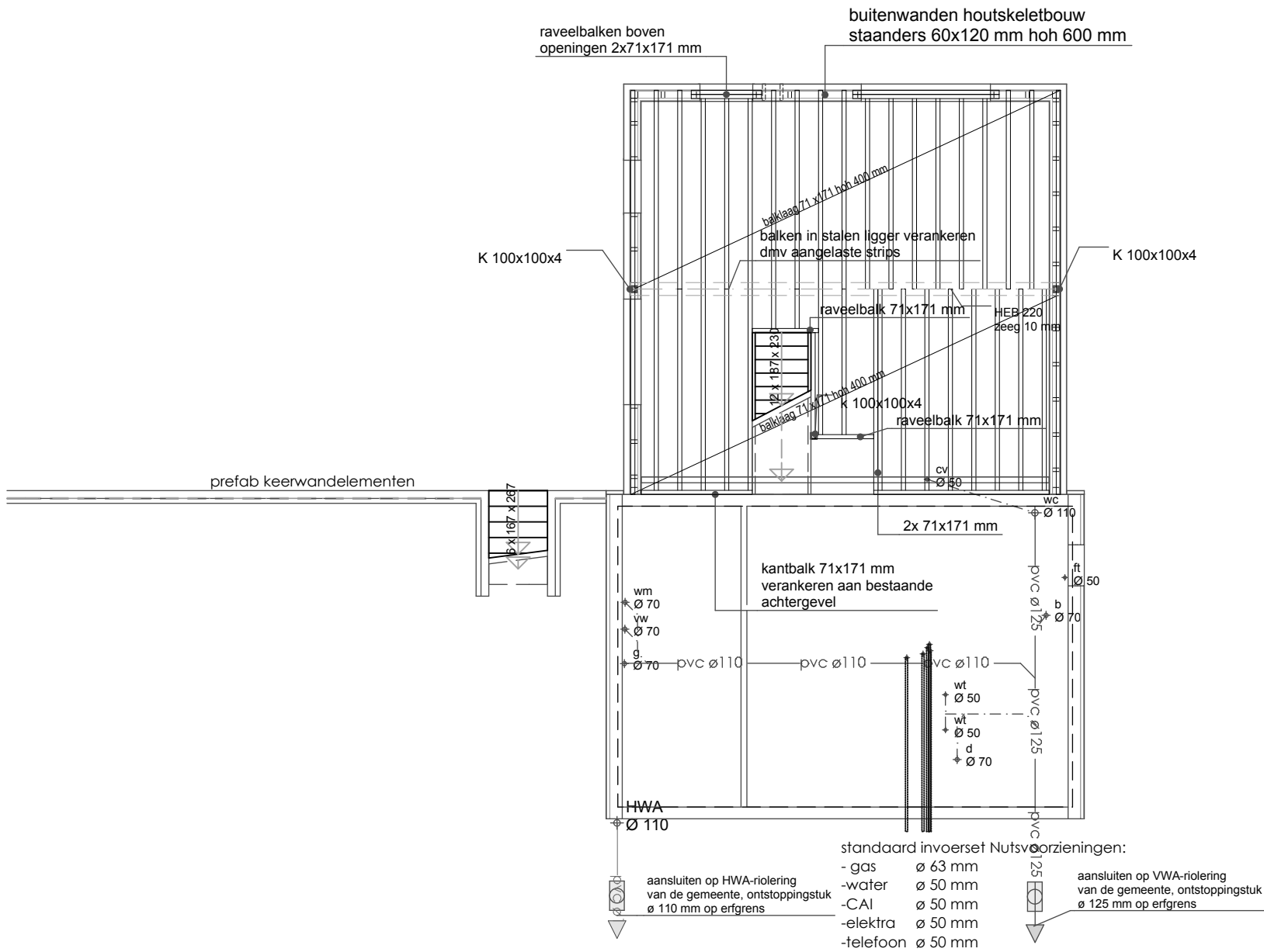
vloer niv 688+
